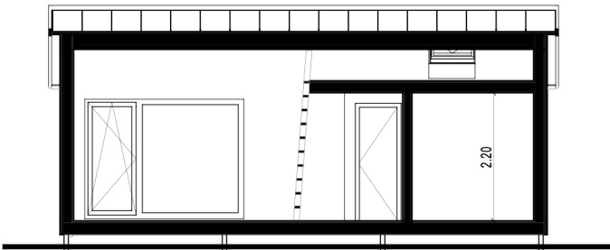
C GRIEZUMS 1:75
