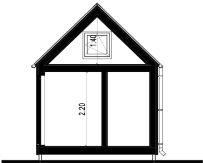
A GRIEZUMS 1:75
