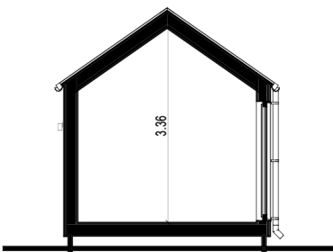
B GRIEZUMS 1:75
