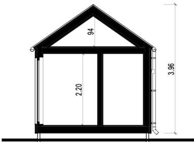
C GRIEZUMS 1:75
