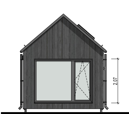
F4 ELEVATION 1:80
